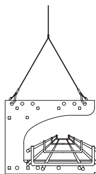
Y-Fit mit Haken, Gripple G-Profil und Kabelrinne
