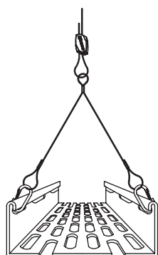
Y-Fit Zubehör mit Karabiner in Kombination mit Gripple HF
