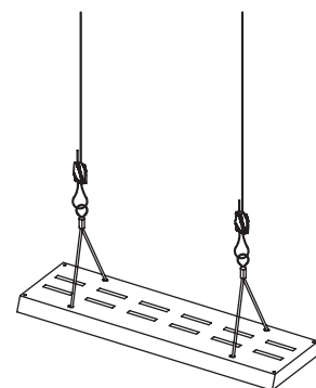
Y-Fit Zubehör an einem Lichtband
