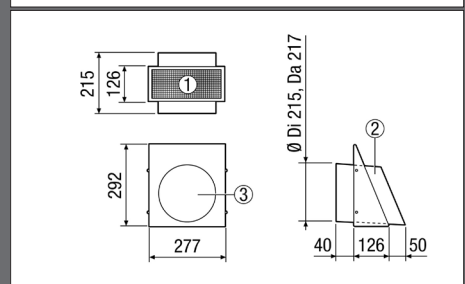
Technische Zeichnung
